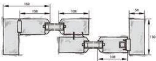
Coupe horizontale
