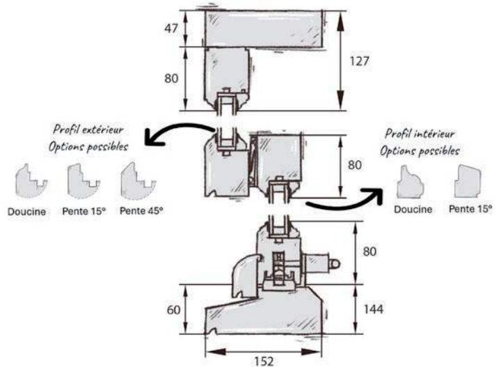
Coupe verticale
