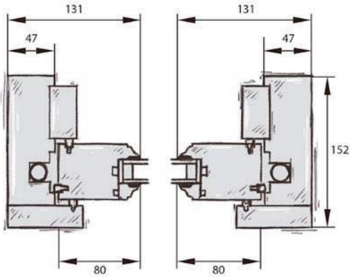
Coupe horizontale
